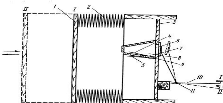
Рисунок 1.3 – Звукообразование в хроматической гармонике: 1 – басовая крышка; 2 – меховая камера; 3 – дека; 4 – язычок внутренний; 5 – язычок наружный; 6 – отверстие в деке; 7 – клапан; 8 – воздушная ось резонатора; 9 – голосовая планка; 10 – клавиша; 11 – ось вращения клавиши 55 .
