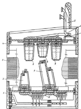
Рис. 18. Поперечный разрез двухрядной гармоники: 1 — базовая крышка; 2 — регулятор аккомпанемента; 2' — мех; 4 — крышка мелодии; 5 — гриф; 6 — рычаги клавиатуры мелодии; 7 — опорные гребенки; 8 — регуляторы мелодии; 9 — регулятор баса; 10 — базовый механизм
